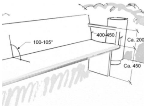
Mynd 9. Bekkur með málsetningum, öll mál í mm
