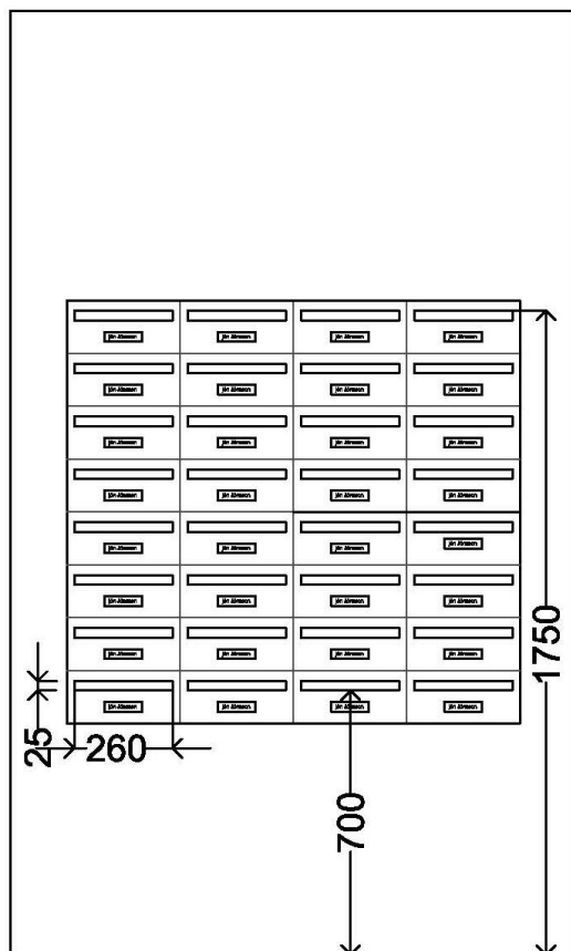
Mynd 2. Bréfastassamstæða, öll mál í mm
