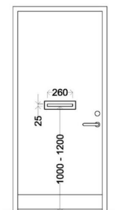
Mynd 1. Bréfarifa á hurð, öll mál í mm
