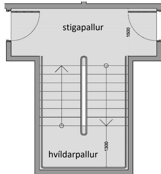
Mynd 4. Dæmi um stigapall þar sem hurð opnast út í stigahús í 2ja hæða íbúðarbyggingu. Öll mál í mm.
