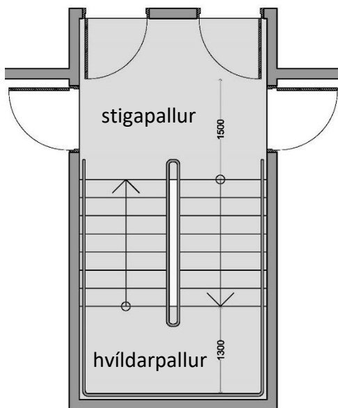
Mynd 5. Dæmi um stigapall þar sem hurð opnast út í stigahús þvert á stigapall í 2ja hæða íbúðarbyggingu. Öll mál í mm.
