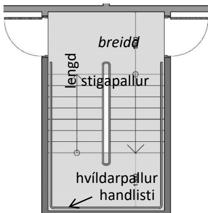
Mynd 1. Dæmi um stigapalla í 2 hæða íbúðarbyggingu. Öll mál í mm.
