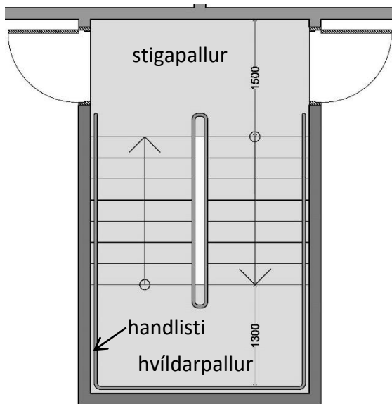
Mynd 3. Dæmi um stigapall þar sem hurð, opnast inn í íbúð í 2ja hæða íbúðarbyggingu. Öll mál í mm.
