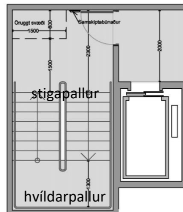
Mynd 2. Dæmi um stigapalla í byggingum með lyftu. Öll mál í mm.
