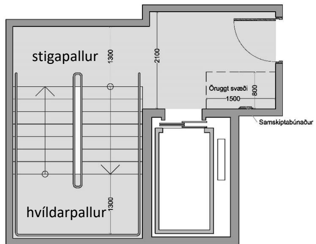
Mynd 6. Dæmi um stigapall þar sem hurð opnast út í stigahús í byggingu með lyftu. Öll mál í mm.
