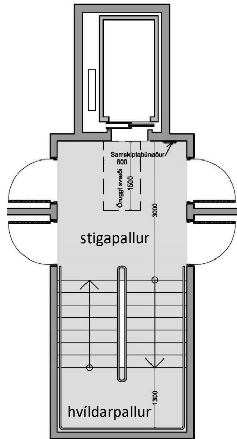
Mynd 8. Dæmi um stigapall í byggingu með lyftu. Öll mál í mm.
