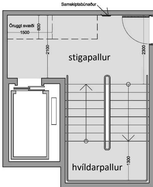
Mynd 7. Dæmi um stigapall þar sem hurð opnast út í stigahús í byggingu með lyftu. Öll mál í mm.
