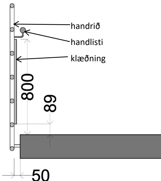
Mynd 4. Sneiðing með dæmi um klæðningu á handriði með láréttum eða hallandi rimlum, öll mál í mm
