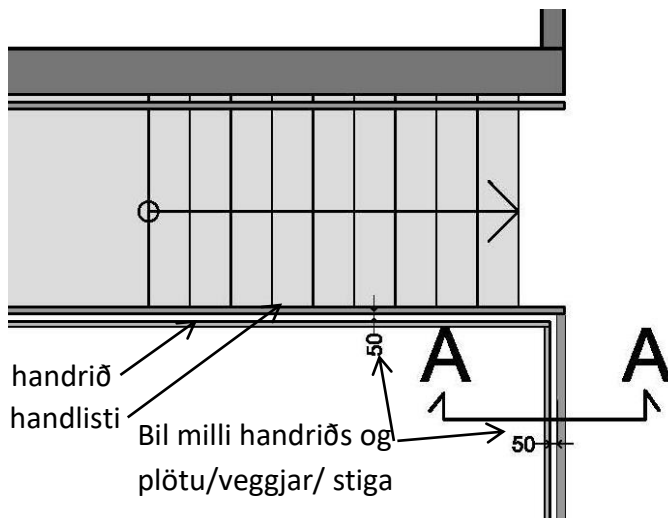
Mynd 2. Dæmi um bil milli utan á liggjandi handriðs og stiga eða svalaplötu
