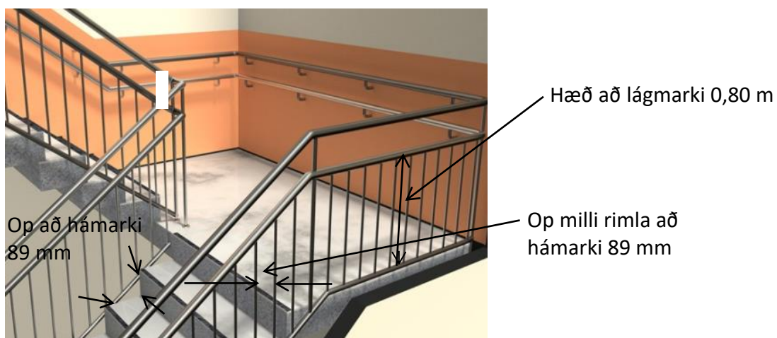
Mynd 1. Dæmi um op í handriði
