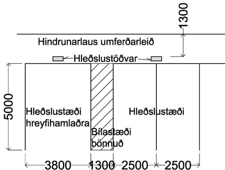
Mynd 1. Gott dæmi um hleðslustöð við bílastæði hreyfihamlaðra. Hleðslustæði hreyfihamlaðra þarf svo að merkja með tákni hreyfihamlaðra á bláum feringi og öll hleðslustæðin með tákni hleðslustæða rafbíla á grænum feringi. Öll mál í mm.
